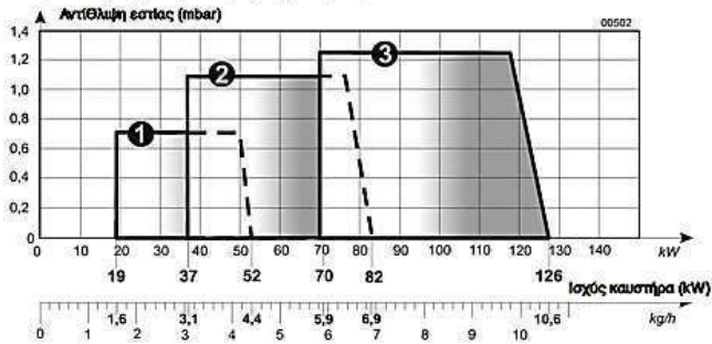
Καμπύλες ισχύος σε υψόμετρο 0 μέτρων
