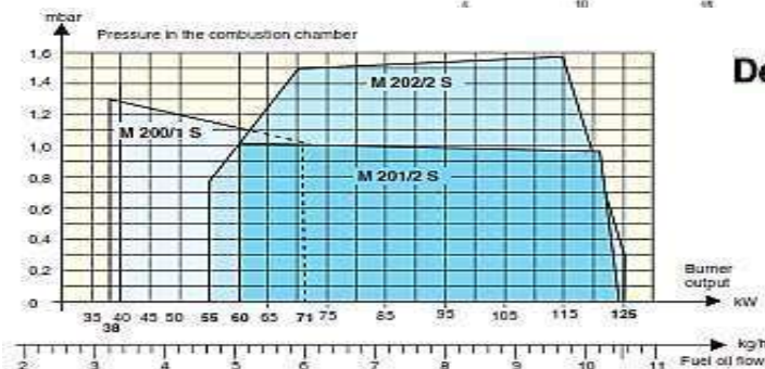
Καμπύλες ισχύος σε υψόμετρο 0 μέτρων
